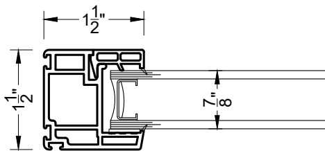
③ JAMB PW215
