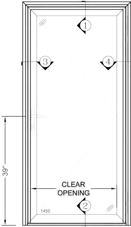
1450 OUT-SWING DOOR
