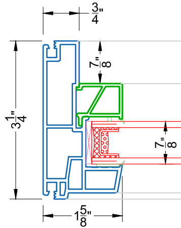
3 JAMB PW 211
