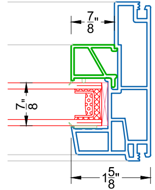
4 JAMB PW 211
